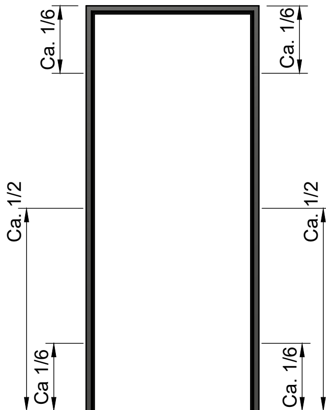
Hullplassering i profil
