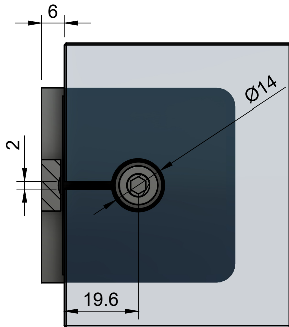
Glass med Ø14 hull og teknisk snitt
